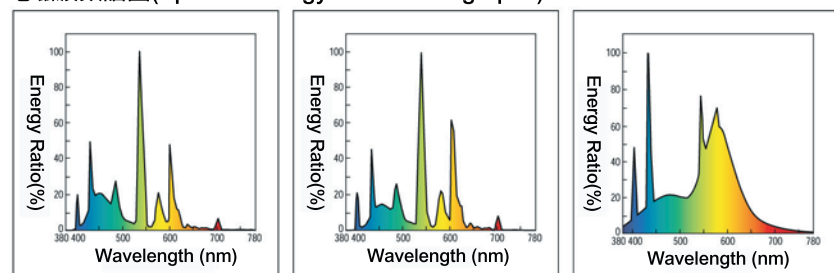
EX-D：三基色白光
